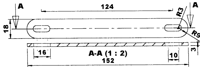
HZ12V200
